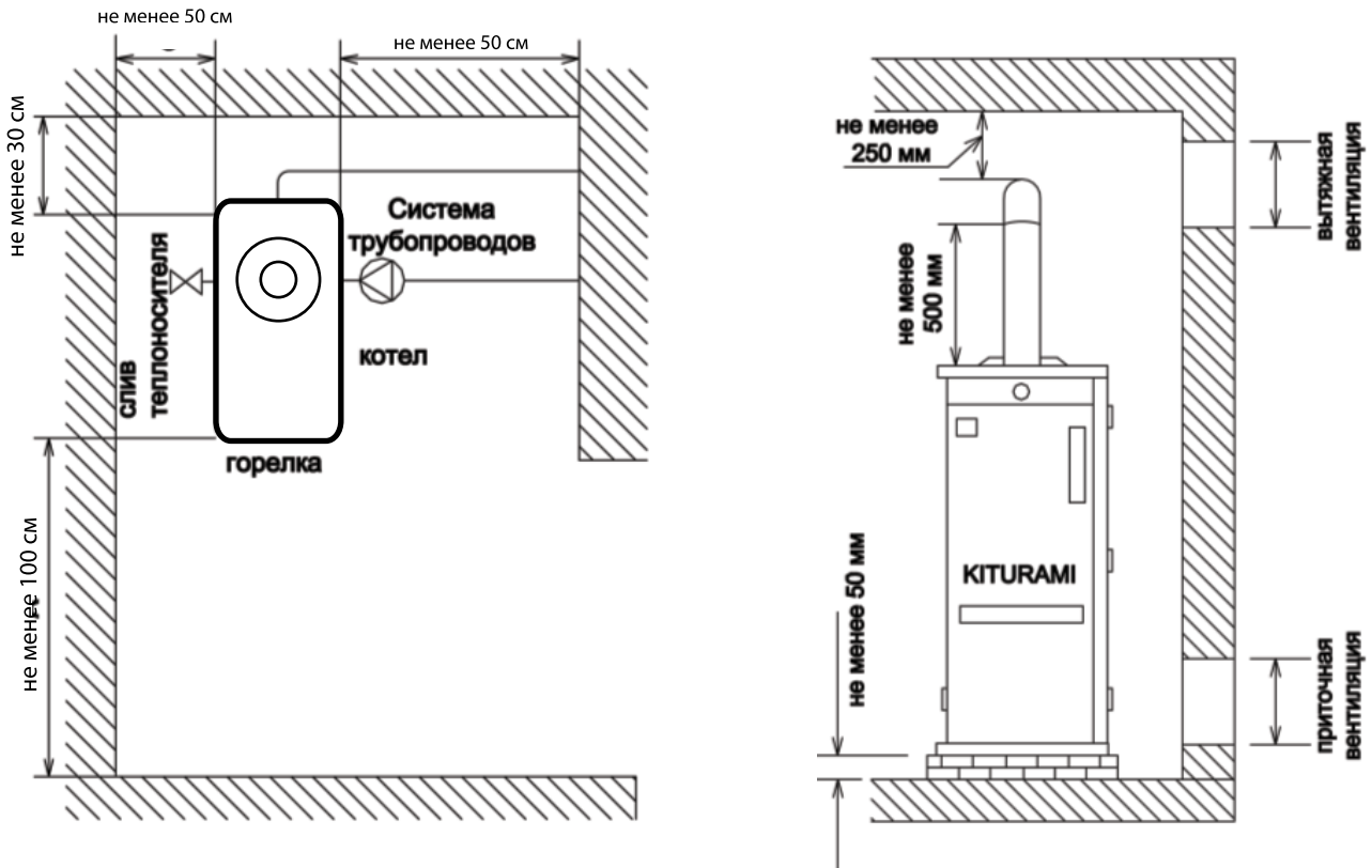
Рисунок 16. Установка котла
