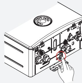
Кнопка аварийного запуска
